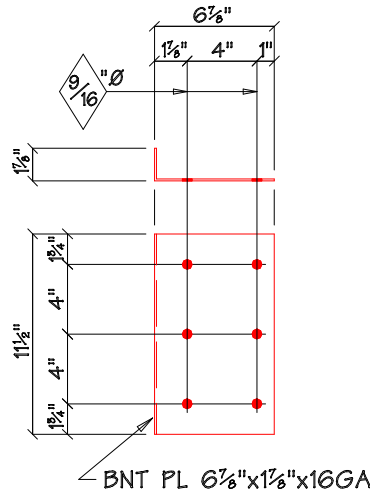
GIRT CLIP~MK P25
