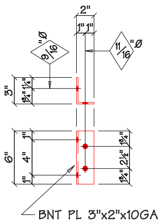
JAMB BASE CLIP~MK P19
