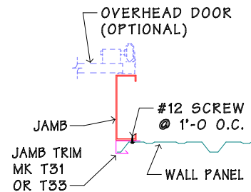
SECTION THRU JAMB
