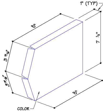
RAKE END CAP - MK T8
